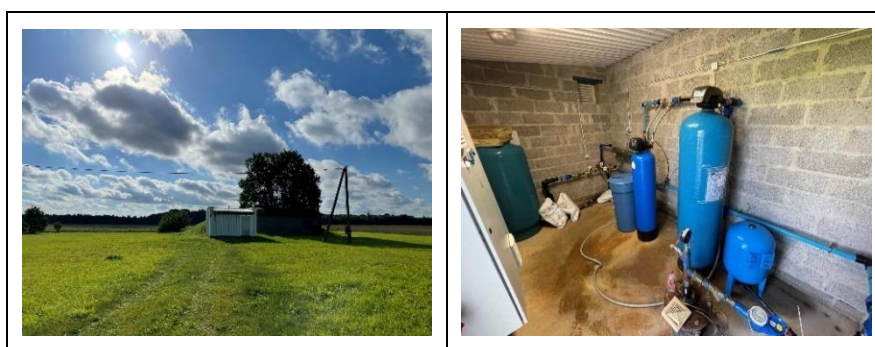
Fotod 4.19 Vägari veetöötlusjaam (2023).
