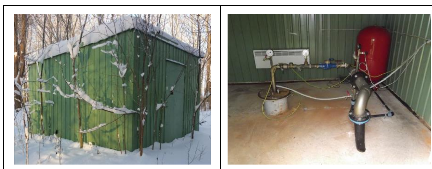
Fotod 4.3 Lillevere puurkaev-pumpla (2023, seest pilt OÜ Alkranel 2013).
