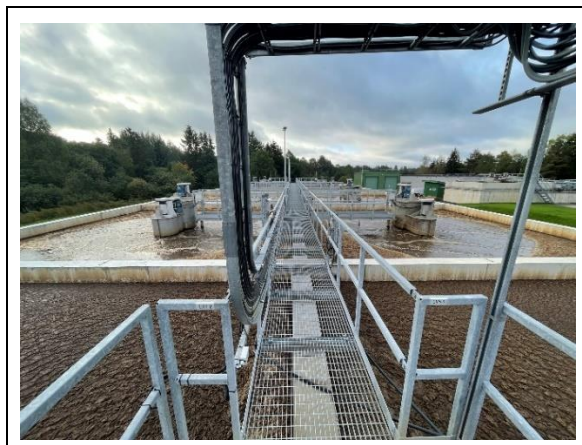
Fotod 5.3 Põltsamaa RVP bioloogilise kompleksi kaks liini (2023).
