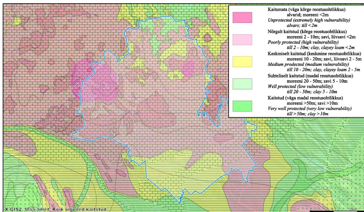
Joonis 2.1 Põltsamaa valla põhjavee kaitstus (Maa-ameti geoportaal).
