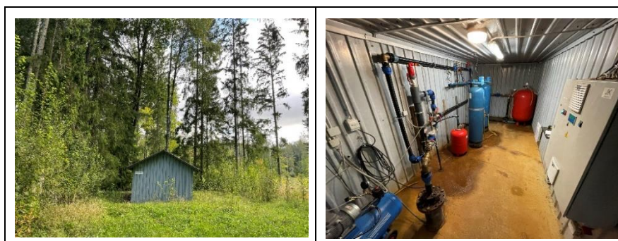
Fotod 4.18 Pisisaare veetötlusjaam ja Kasevõsa PRK (2023).
