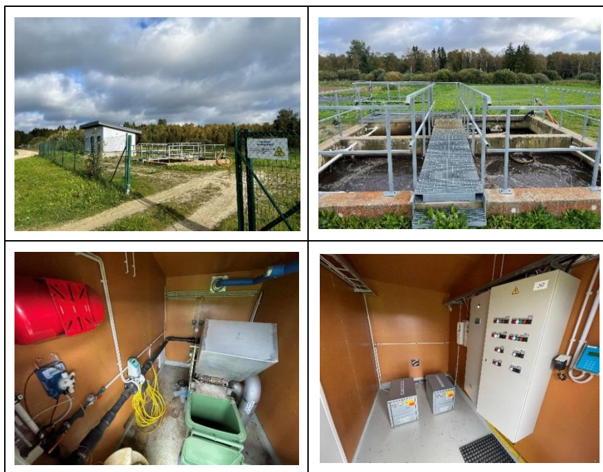
Fotod 5.11 Põltsamaa reoveepuhasti ja biotiigid (2023).
