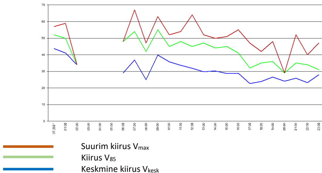
Diagrammil 2.2 Sõidukiirused Kuuse tänaval tööpäeval
