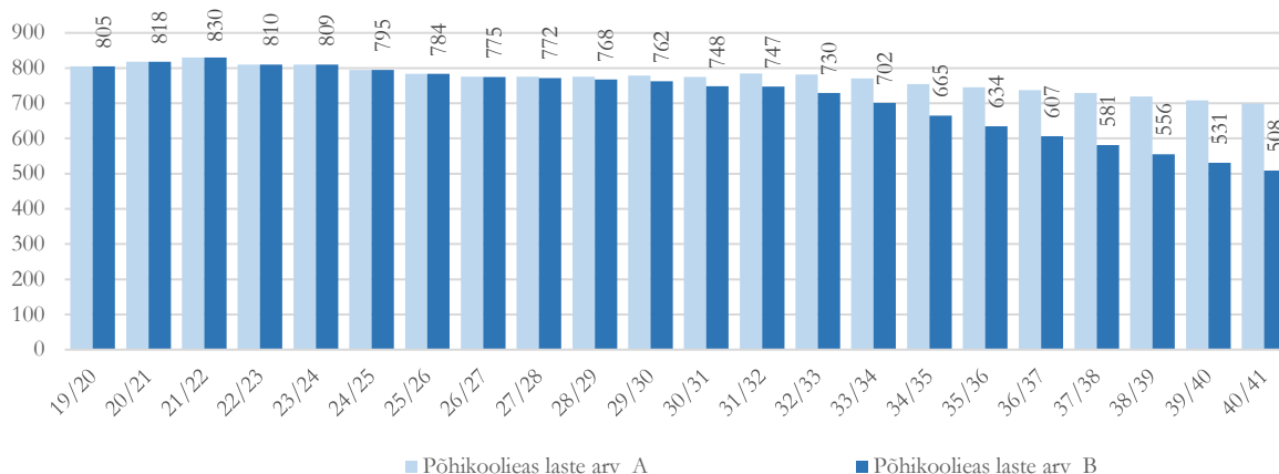
Joonis 20. Põhikoolieas laste arvu prognoos Põltsamaa vallas aastani 2040
