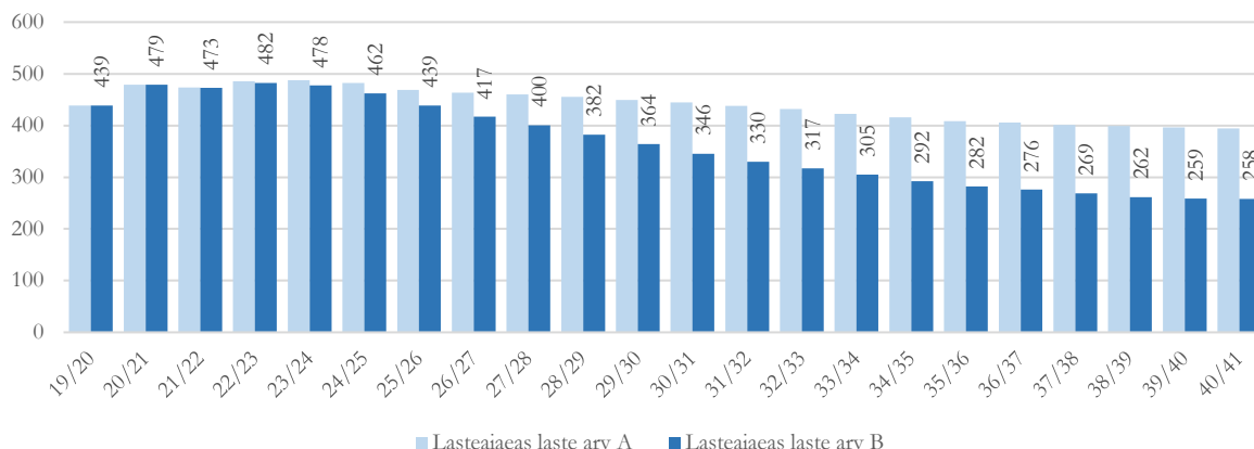
Joonis 19. Lasteiaegas laste arvu prognoos Põltsamaa vallas aastani 2040
