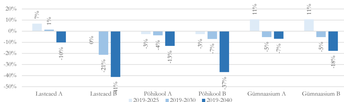
Joonis 18. Lasteaia-, põhikooli- ja gümnaasiumieas laste arvu muutuse prognoos Põltsamaa vallas aastani 2040
