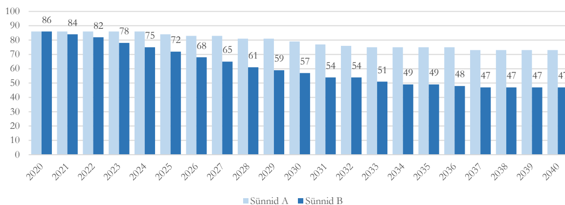
Joonis 17. Põltsamaa valla sündide arvuprognos aastani 2040
