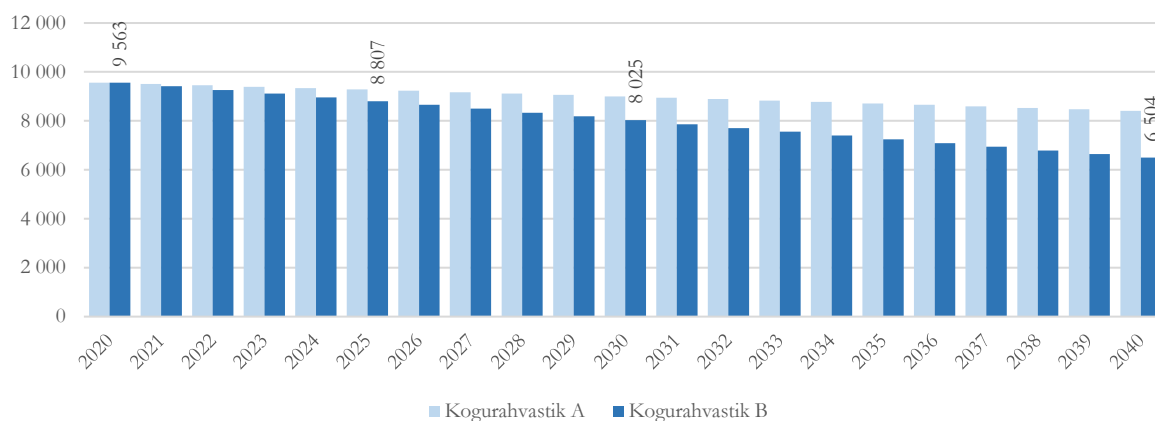
Joonis 16. Põltsamaa valla kogurahvastiku prognoos aastani 2040 2
