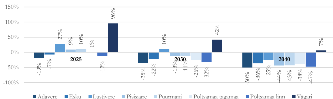
Joonis 23. Lasteaia laste arvu muutuse prognoos piirkondades aastani 2040 (rände-stsenaarium)
