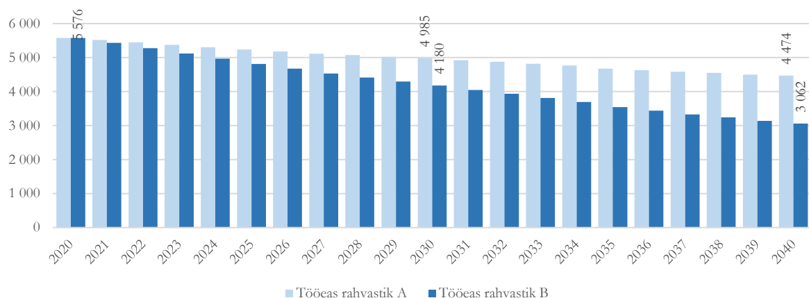
Joonis 26. Tööeas elanike (vanus 19-64) arvu prognoos Põltsamaa vallas aastani 2040
