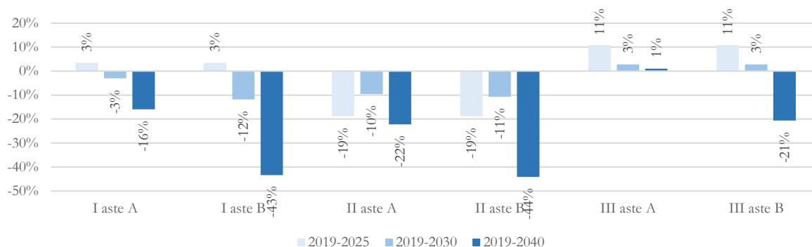
Joonis 21. Põhikoolieas laste arvu prognoos kooliastmete lõikes Põltsamaa vallas aastani 2040
