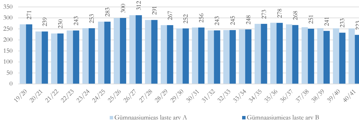
Joonis 22. Gümnaasiumieas laste arvu prognoos Põltsamaa vallas aastani 2040
