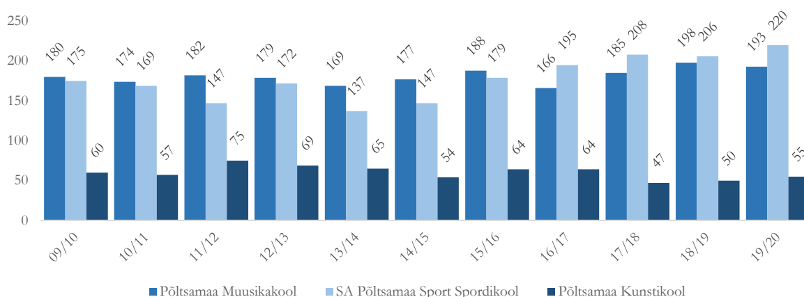
Joonis 34. Õpilaste arv huvikoolides õppeaastatel 09/10 kuni 19/20 (EHIS)
