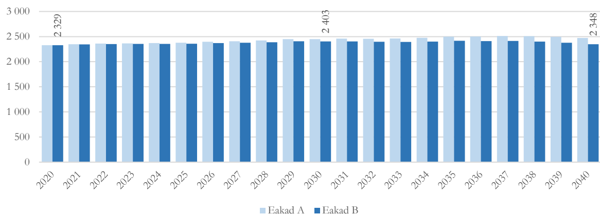
Joonis 27. Eakate (vanus 65+) arvu prognoos Põltsamaa vallas aastani 2040
