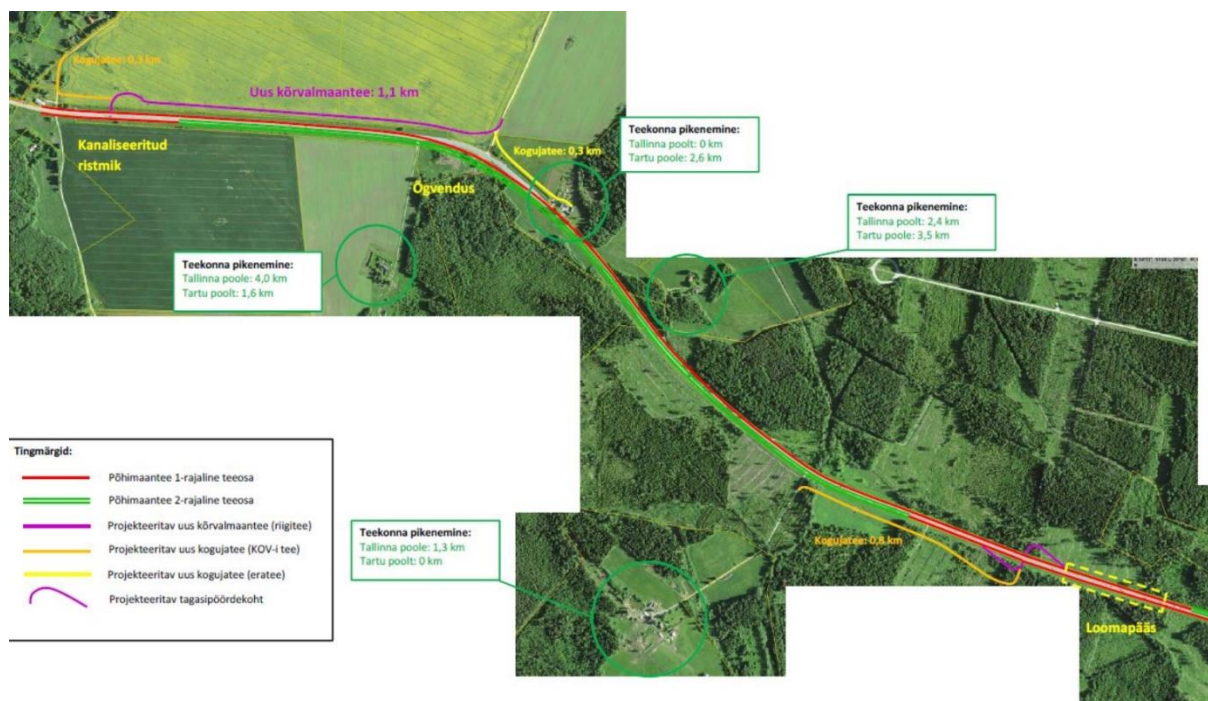
Joonis 7. Kavandatav Neanurme-Pikknurme 2+1 projektlahendus. Allikas: Maanteeamet 3
